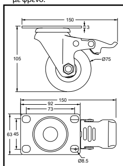
Διαστάσεις μικρής ρόδας Υ. 105 με φρένο.
