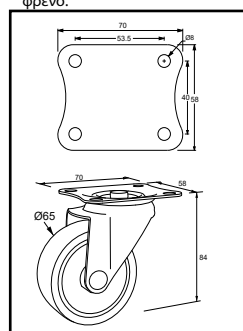
Διαστάσεις ρόδας Υ. 84 χωρίς φρένο.
