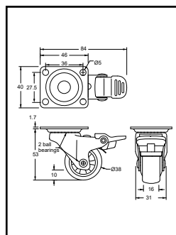
Διαστάσεις μικρής ρόδας Υ. 53 με φρένο.
