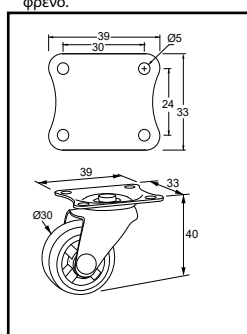
Διαστάσεις ρόδας Υ. 40 χωρίς φρένο.
