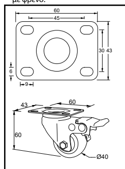
Διαστάσεις μικρής ρόδας Υ. 60 με φρένο.
