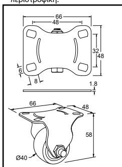
Διαστάσεις ρόδας Υ. 5.8, μη περιστροφική.
