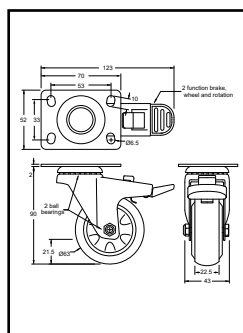
Διαστάσεις μεγάλης ρόδας Υ. 90 με φρένο.
