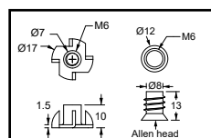
Μπουσουλές στερέωσης [2] για σπείρωμα M6.
