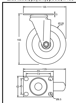
Διαστάσεις μεγάλης ρόδας Υ. 155
