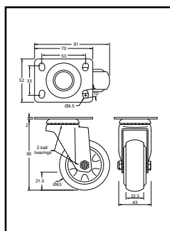
Διαστάσεις μεγάλης ρόδας Υ. 90 χωρίς φρένο.
