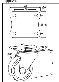
Διαστάσεις ρόδας Υ. 51 χωρίς φρένο.
