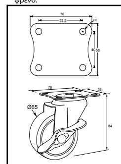
Διαστάσεις ρόδας Υ. 84 με φρένο.
