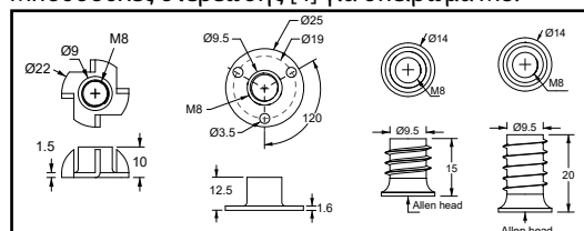
Μπουσουλές στερέωσης [4] για σπείρωμα M8.
