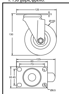
Διαστάσεις μεγάλης ρόδας Υ. 130 χωρίς φρένο.
