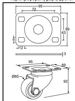
Διαστάσεις ρόδας Υ. 9.2, περιστρεφόμενη χωρίς φρένο.
