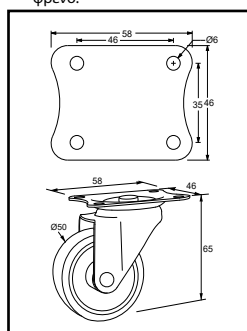
Διαστάσεις ρόδας Υ. 65 χωρίς φρένο.
