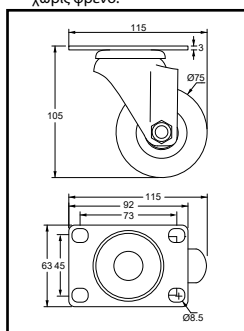
Διαστάσεις μικρής ρόδας Υ. 105 χωρίς φρένο.
