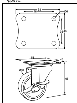
Διαστάσεις ρόδας Υ. 65 με φρένο.
