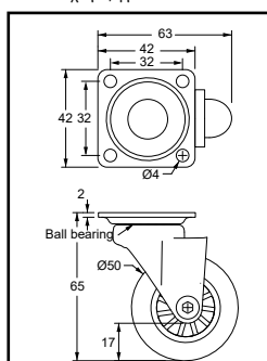
Διαστάσεις μικρής ρόδας Υ. 65 χωρίς φρένο.
