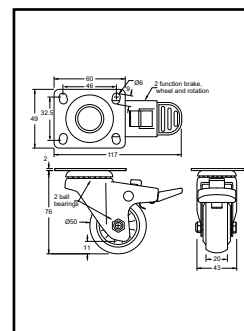
Διαστάσεις μεγάλης ρόδας Υ. 76 με φρένο.
