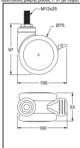
Διαστάσεις μικρής ρόδας Υ. 97 με πείρο.
