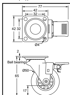
Διαστάσεις μικρής ρόδας Υ. 65 με φρένο.
