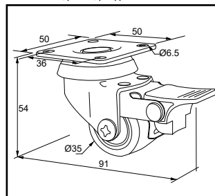
Διαστάσεις ρόδας με φρένο.
