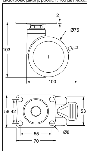
Διαστάσεις μικρής ρόδας Υ. 103 με πλάκα.
