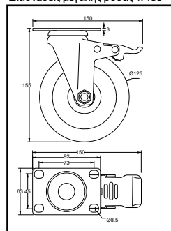
Διαστάσεις μεγάλης ρόδας Υ. 155
