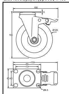
Διαστάσεις μεγάλης ρόδας Υ. 155 με φρένο
