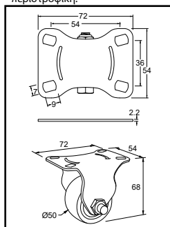
Διαστάσεις ρόδας Υ. 6.8, μη περιστροφική.
