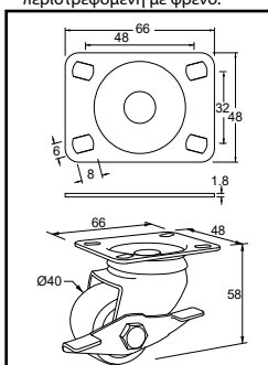
Διαστάσεις ρόδας Υ. 5.8, περιστρεφόμενη με φρένο.
