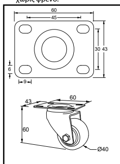
Διαστάσεις μικρής ρόδας Υ. 60 χωρίς φρένο.
