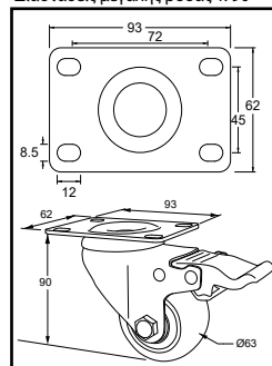
Διαστάσεις μεγάλης ρόδας Υ. 90
