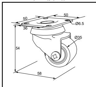
Διαστάσεις ρόδας χωρίς φρένο.
