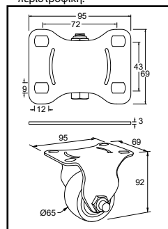
Διαστάσεις ρόδας Υ. 9.2, μη περιστροφική.
