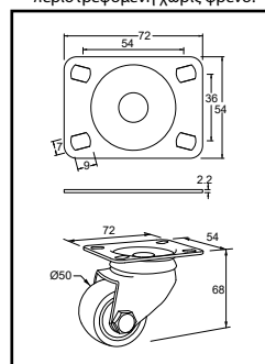
Διαστάσεις ρόδας Υ. 6.8, περιστρεφόμενη χωρίς φρένο.
