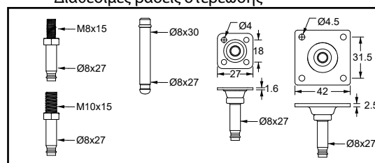
Διαθέσιμες βάσεις στερέωσης
