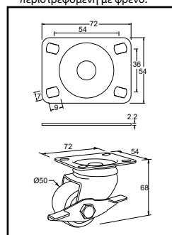
Διαστάσεις ρόδας Υ. 6.8, περιστρεφόμενη με φρένο.
