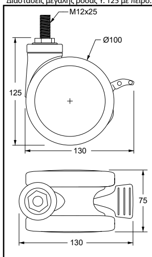
Διαστάσεις μεγάλης ρόδας Υ. 125 με πείρο.
