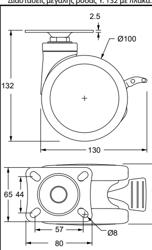
Διαστάσεις μεγάλης ρόδας Υ. 132 με πλάκα.
