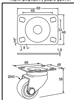
Διαστάσεις ρόδας Υ. 5.8, περιστρεφόμενη χωρίς φρένο.
