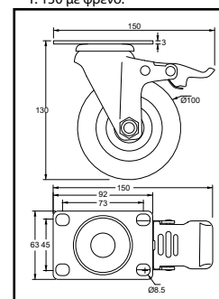
Διαστάσεις μεγάλης ρόδας Υ. 130 με φρένο.
