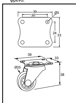
Διαστάσεις ρόδας Υ. 38 χωρίς φρένο.
