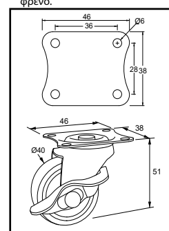
Διαστάσεις ρόδας Υ. 51 με φρένο.
