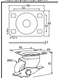
Διαστάσεις ρόδας Υ. 9.2, περιστρεφόμενη με φρένο.
