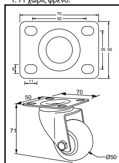
Διαστάσεις μεγάλης ρόδας Υ. 71 χωρίς φρένο.
