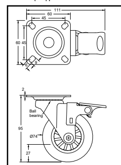
Διαστάσεις μεγάλης ρόδας Υ. 95 με φρένο.
