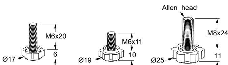
Μπουσουλές στερέωσης [2] για σπείρωμα M6.
