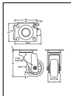
Διαστάσεις μεγάλης ρόδας Υ. 76 χωρίς φρένο.
