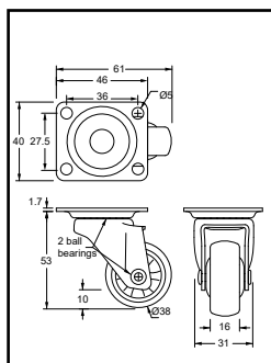
Διαστάσεις μικρής ρόδας Υ. 53 χωρίς φρένο.
