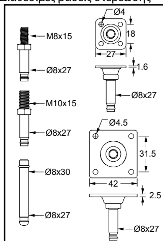
Διαθέσιμες βάσεις στερέωσης
