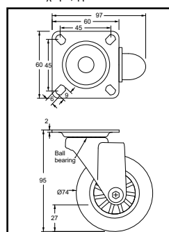
Διαστάσεις μεγάλης ρόδας Υ. 95 χωρίς φρένο.
