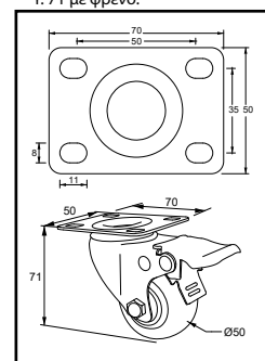
Διαστάσεις μεγάλης ρόδας Υ. 71 με φρένο.
